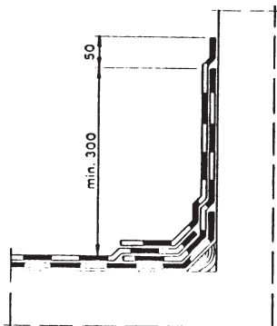
Kuva 8. Seinällenosto, 2-kermikate.
