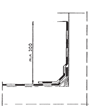
Kuva 7. Seinällenosto, 1-kermikate.
