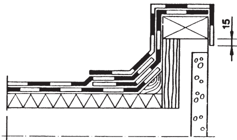
Kuva 5. Räystäs, 2-kermikate.
