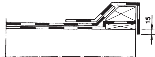
Kuva 1. Saneeraustyö, korotettu räystääs, 1-kermikate.
