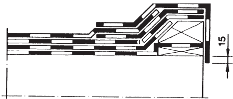
Kuva 3. Saneeraustyö, korotettu räystäs, 3-kermikate.
