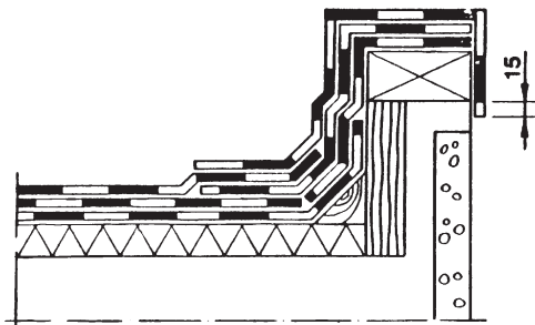
Kuva 6. Rästäs, 3-kermikate.
