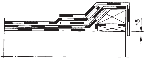
Kuva 2. Saneeraustyö, korotettu räystääs, 2-kermikate.
