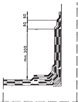
Kuva 9. Seinällenosto, 3-kermikate.
