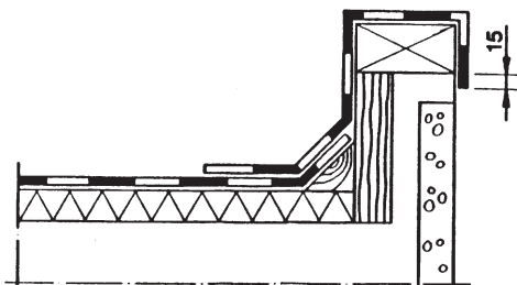
Kuva 4. Räystäs, 1-kermikate.
