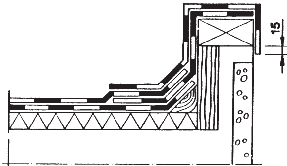
Kuva 5. Räystäs, 2-kermikate.
