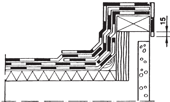
Kuva 6. Rästäs, 3-kermikate.
