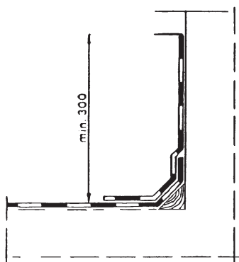
Kuva 7. Seinällenosto, 1-kermikate.
