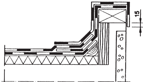
Kuva 5. Räystäs, 2-kermikate.
