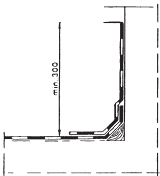
Kuva 7. Seinällenosto, 1-kermikate.
