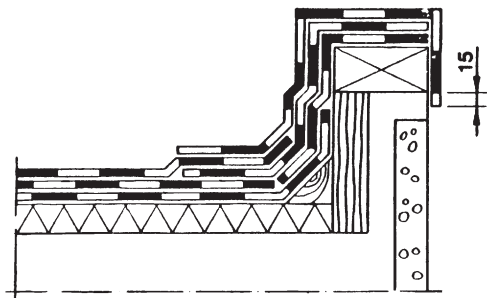
Kuva 6. Rästäs, 3-kermikate.
