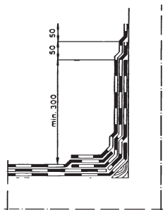
Kuva 9. Seinällennosto, 3-kermikate.
