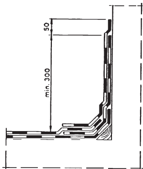
Kuva 8. Seinällenosto, 2-kermikate.
