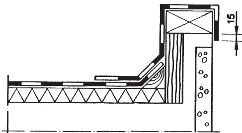
Kuva 4. Räystäs, 1-kermikate.
