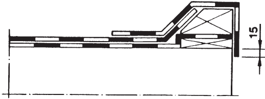
Kuva 1. Saneeraustyö, korotettu räystäs, 1-kermikate.
