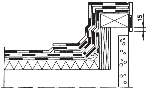
Kuva 6. Räystäs, 3-kermikate.
