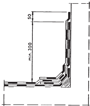
Kuva 8. Seinälienosto, 2-kermikate.
