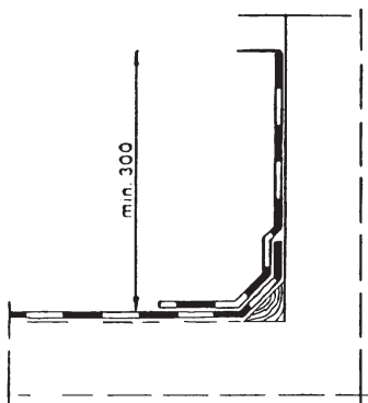
Kuva 7. Seinälienosto, 1-kermikate.
