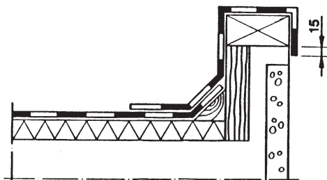
Kuva 4. Räystäs, 1-kermikate.
