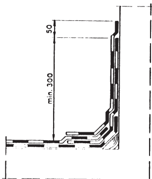
Kuva 8. Seinällenosto, 2-kermikate.
