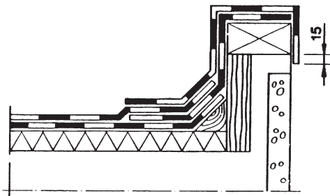
Kuva 5. Räystäs, 2-kermikate.
