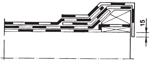
Kuva 2. Saneeraustyö, korotettu räystäs, 2-kermikate.
