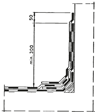
Kuva 8. Seinäliennosto, 2-kermikate.
