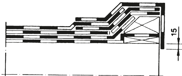
Kuva 3. Saneeraustyö, korotettu räystäs, 3-kermikate.
