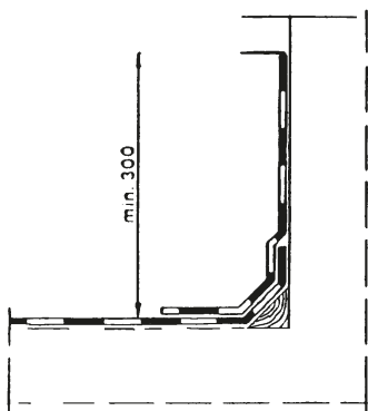
Kuva 7. Seinäliennosto, 1-kermikate.
