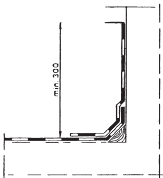
Kuva 7. Seinällenosto, 1-kermikate.
