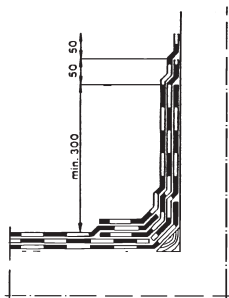
Kuva 9. Seinällennosto, 3-kermikate.
