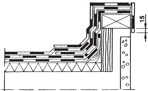
Kuva 6. Rästäs, 3-kermikate.
