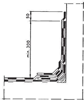
Kuva 8. Seinällenosto, 2-kermikate.
